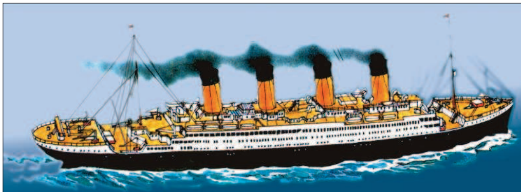
Корабль «Титаник»
