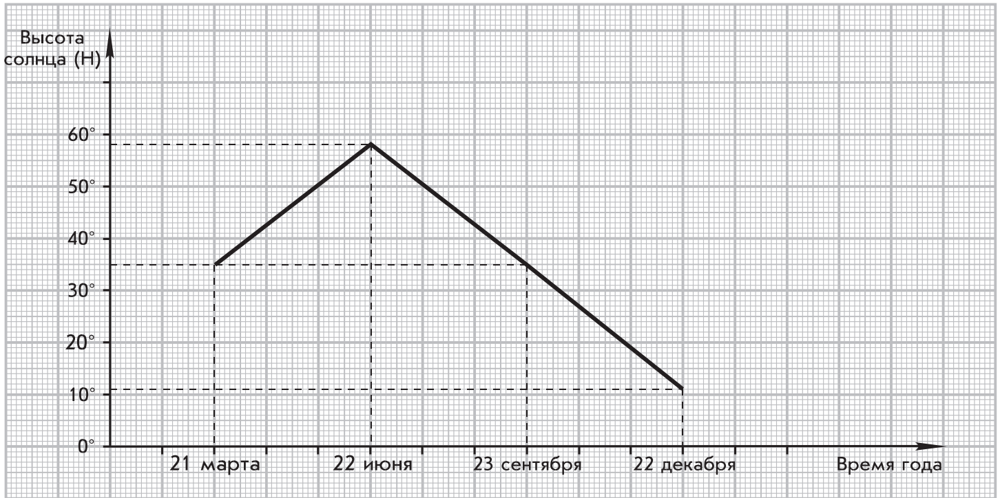
Рис. 2. График годового изменения высоты солнца над горизонтом на широте Москвы
