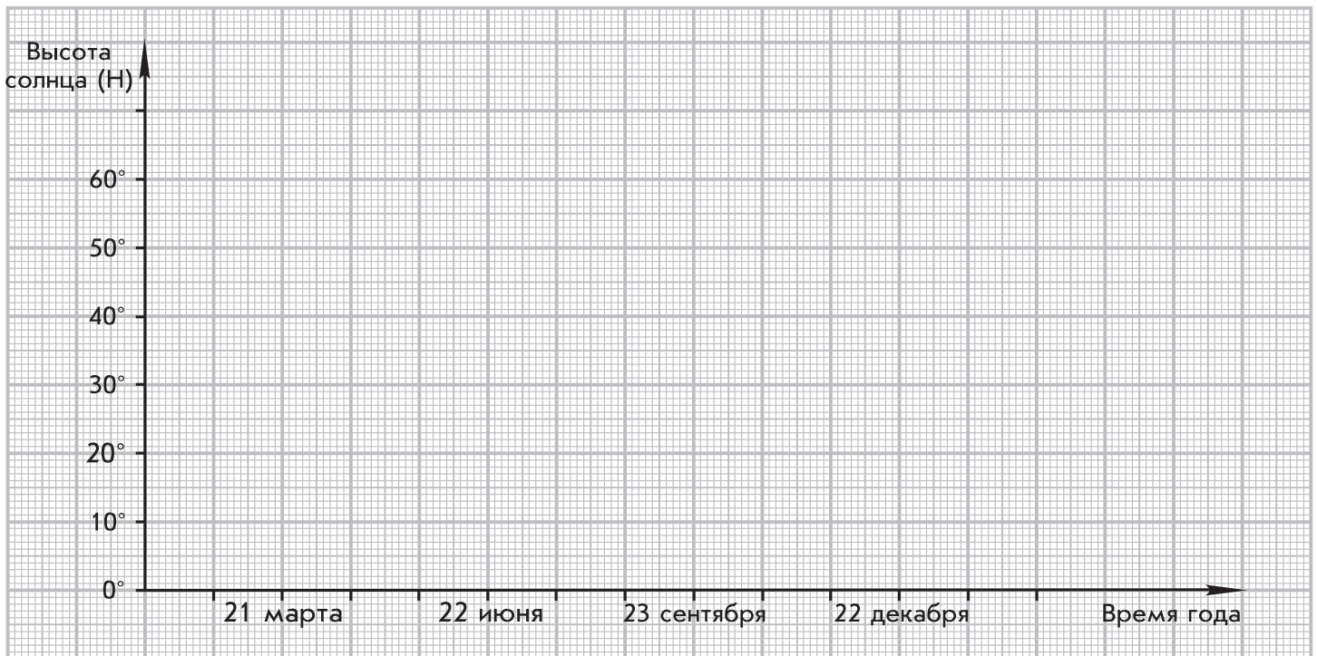
Рис. 3. График годового изменения высоты солнца над горизонтом на широте своего населённого пункта
